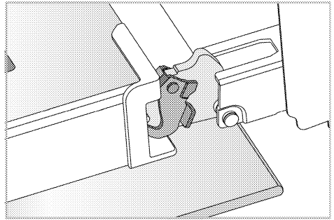
Hængselås - åben position
