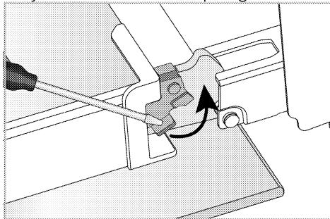
Hængselås - lukket position
