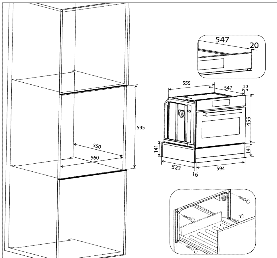
Wärmeschublade unter einem 45 cm Kompaktofen in einer Turmeinheit
